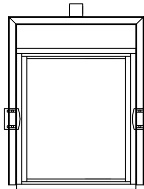
Parte movil (elevador)
